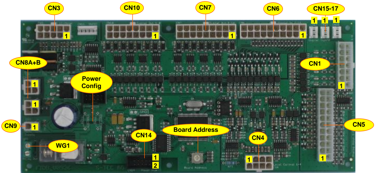
Abbildung 1: Universelle-IOKarte FIOB V0936
