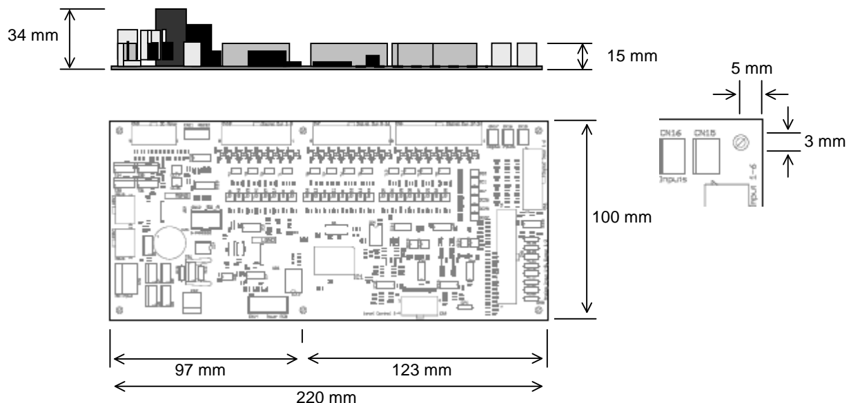
Abbildung 3: Abmessungen der universellen I/O-Karte FIOB (Aufriss, Grundriss und Lochmasse)
