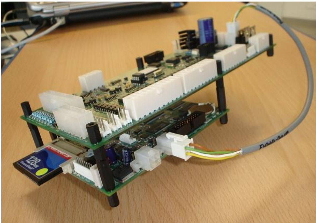
Abbildung 2: Huckepack-Montage mit dem eigerPanel 57
