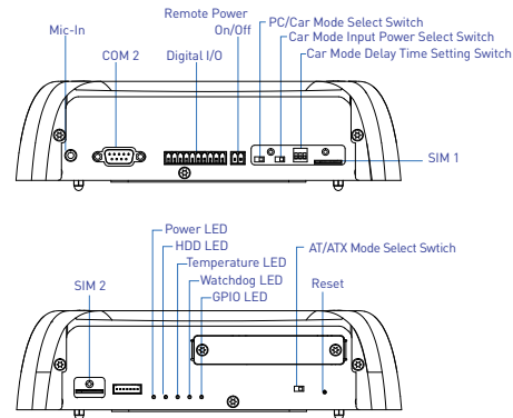
Left I/O
