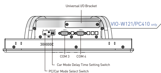
Right I/O
