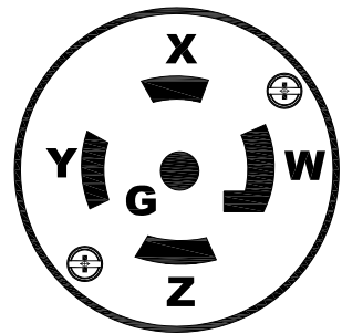
NEMA L22-30P
