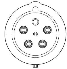
IEC60309 63A 3PY
