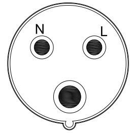
IEC60309 63A 3P
